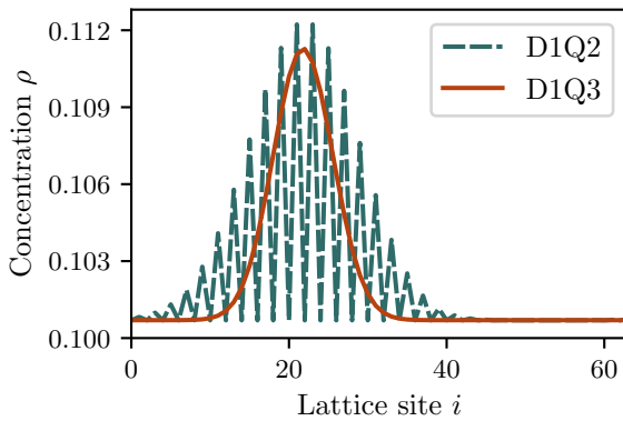
(a) D1Q2 and D1Q3
